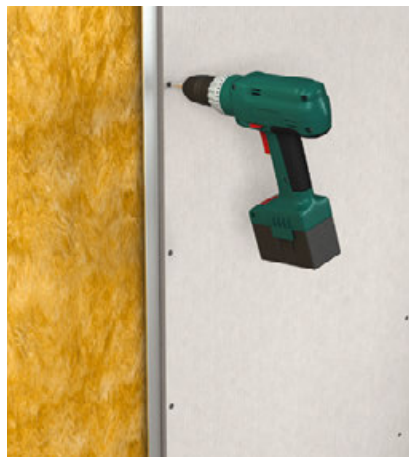
Befestigung mit Schrauben
