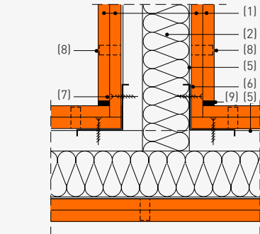
Wandverbindung in T-Form mit unterbrochener Längsflanke und LW-Inneneckprofil
