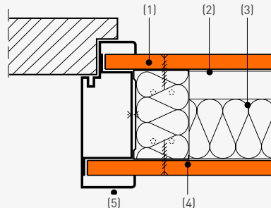
Zargenbefestigung direkt an CW-Profilen
