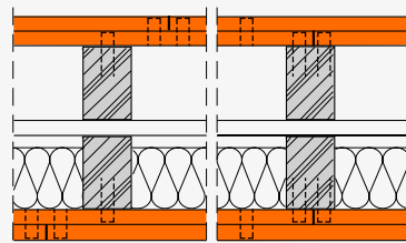
Montagewand mit fermacell® Gipsfaser-Platten mit Hohlraum­dämmung als Doppelständerwand, doppel­lagig bekleidet
