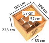
PEPE 2 MIT ANBAUDACH ▶ Seite 76
