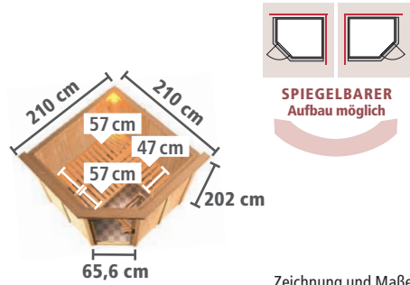
Zeichnung und Maße mit Dachkranz
