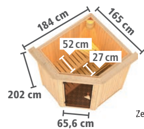
Abb. TONJA mit Dachkranz und Zubehör (gegen Aufpreis): Saunaleuchte Premium und Bodenrost
