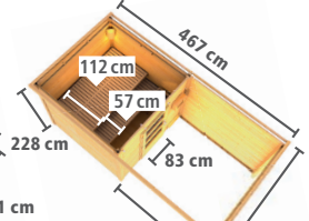
PEPE 4 MIT ANBAUDACH ▶ Seite 77
