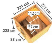
PEPE 4 MIT ANBAUDACH ▶ Seite 77
